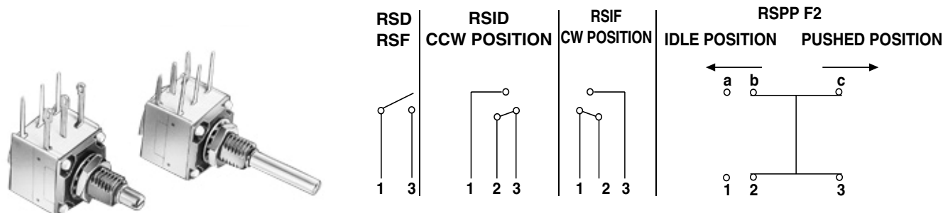
SWITCH MODULES
